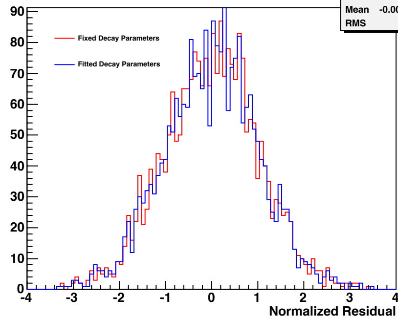
sum91-2-1_sum591-1_21-1_michel.root
