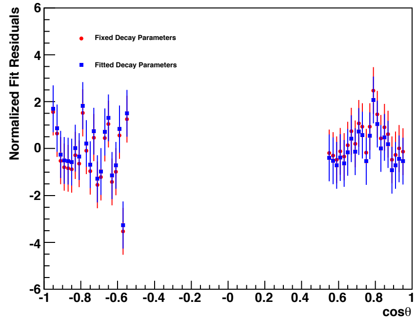
sum93-2-1_sum593-1_21-1_michel.root
