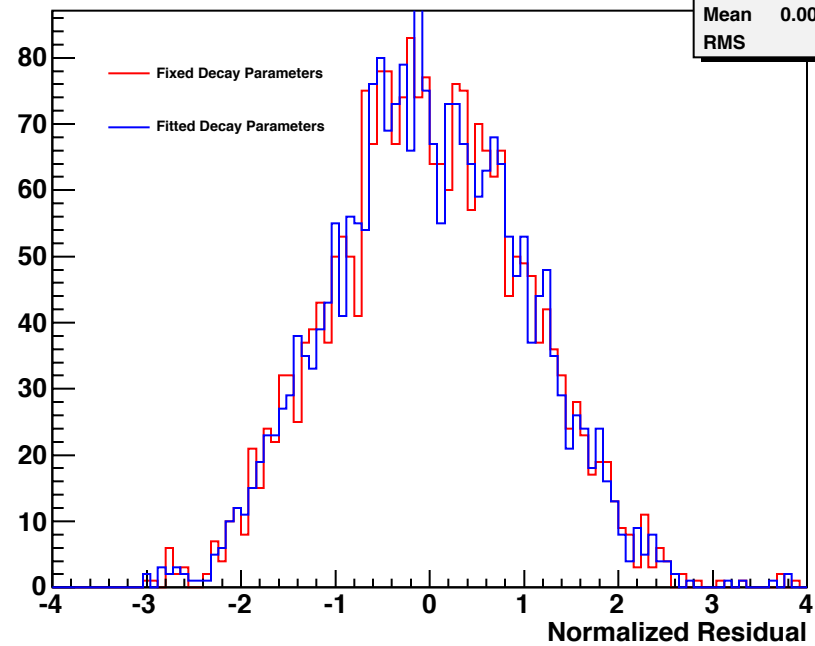
sum93-2-1_sum593-1_21-1_michel.root
