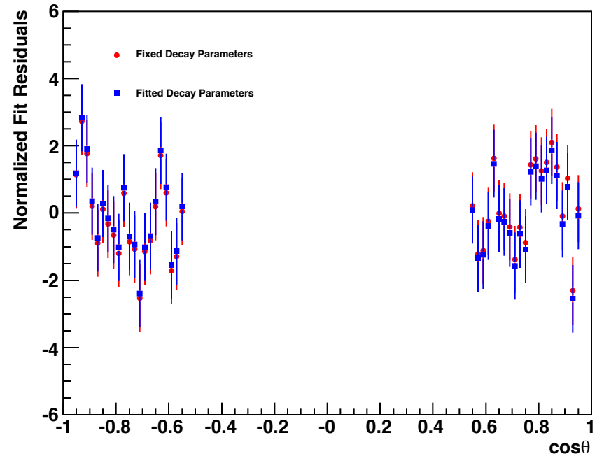
sum84-9-1_sum584-1_2_21-1_michel.root
