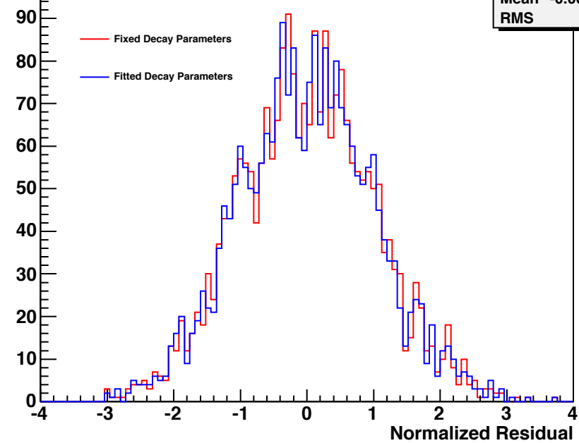
sum84-9-1_sum584-1_2_21-1_michel.root
