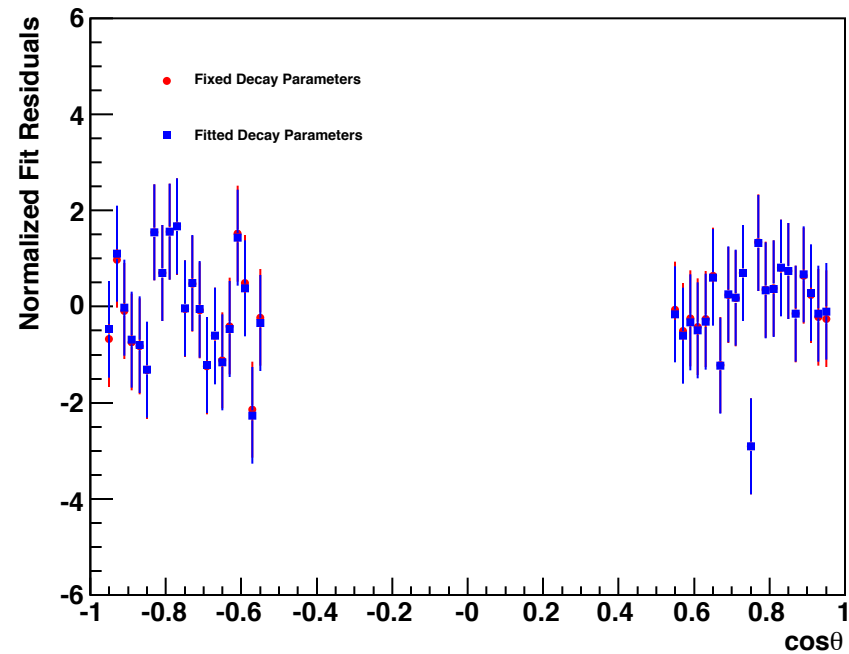
sum91-2-1_sum591-1_21-1_michel.root
